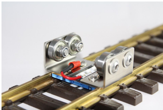
Rollenprüfstand einzeln mit LED 01-02-00
